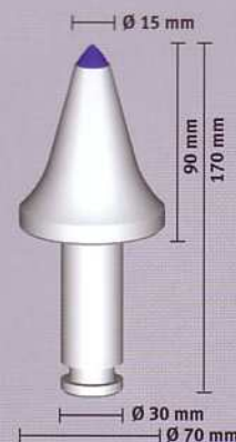
Burin ER 15/90/70/30 Q N° de pièce 19 90 70 35
