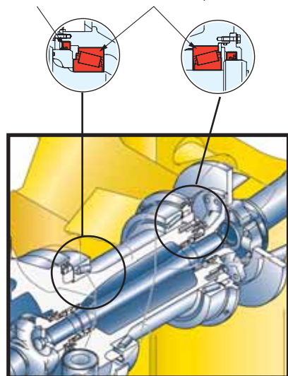
Joint à lèvres Roulements coniques
